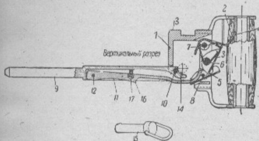
Рис. 11. Затыльник с направляющим стержнем возвратно-боевой пружины:
