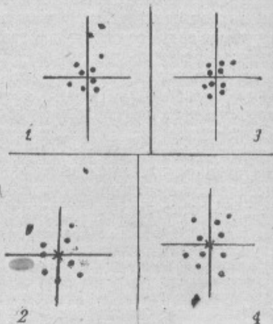
Рис. 30. Определение средней точки попадания по десяти пробойнам
