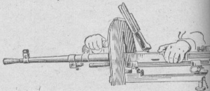
Рис. 27. Отделение ствола от ствольной коробки
