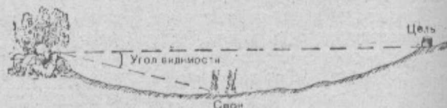
Рис. 41. Измерение угла видимости с помощью бинокля
