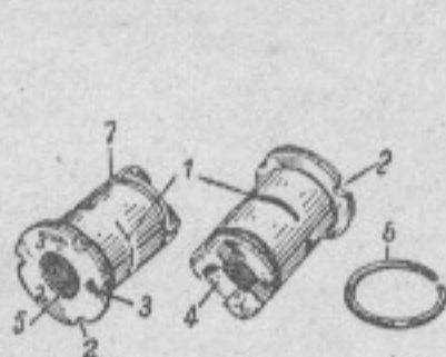
Рис. 4. Регулятор:
