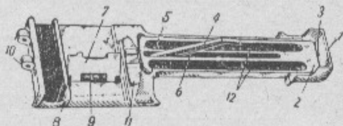
Рис. 15. Крышка приемника:
