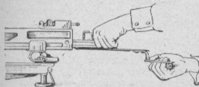
Рис. 26. Вынимание рамы с затвором из ствольной коробки
