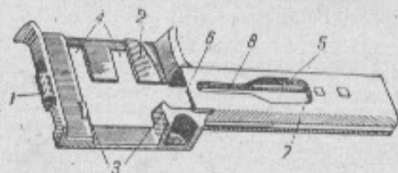
Рис. 12. Основание приемника:
