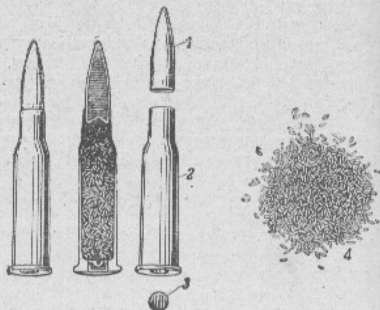
Рис. 23. Боевой патрон:
