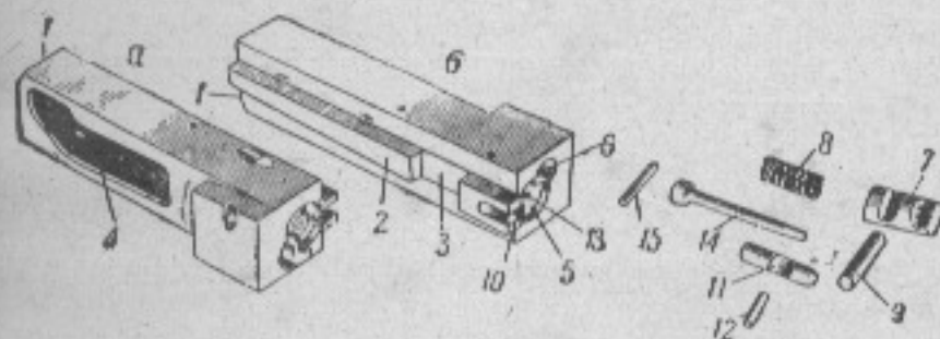
Рис. 9. Затвор:
