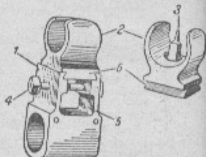
Рис. 5. Основание мушки с предохранителем и мушкой: 1 — основание мушки; 2 — предохранитель мушки; 3 — мушка; 4 — крепительный болт; 5 — стенка основания; 6 — площадка предохранителя мушки
