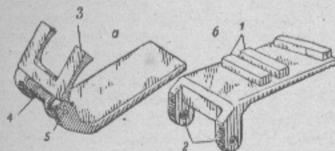
Рис. 16. Ползун с пальцами подачи:
