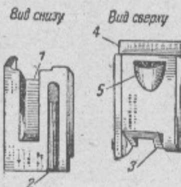
Рис. 17. Замыкатель ствола:
