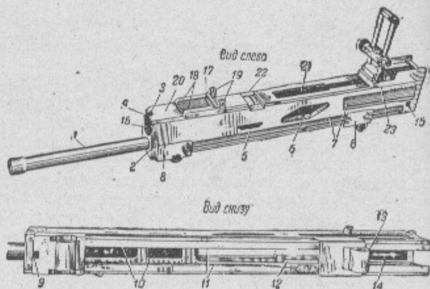
Рис. 6. Ствольная коробка:
