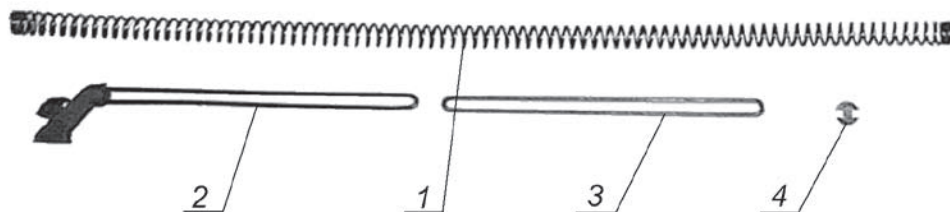
Rys. 63. Urządzenie powrotne:
