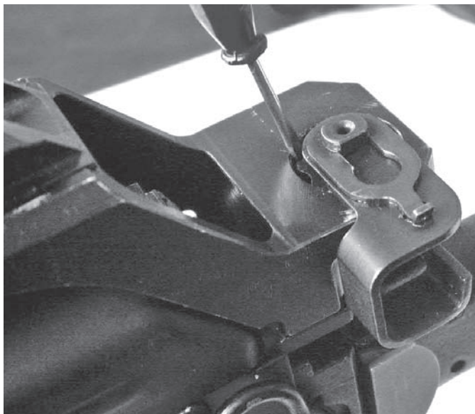
Rys. 38. Zatrzask mimośrodowy w pozycji otwartej – regulacja nakrętki specjalnej zacisku
